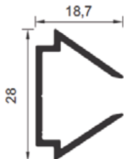
FCX-0207 BAGUETE VIDRO
