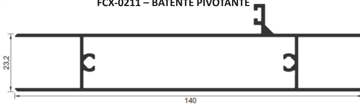
FCX-0211 – BATENTE PIVOTANTE
