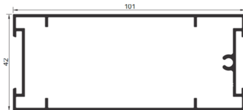
FCX-0219 – MONTANTE PIVOTANTE
