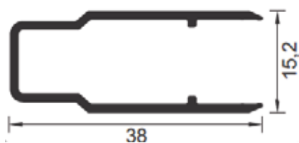
FCX-0209 MINI LAMBRI - DETALHE
