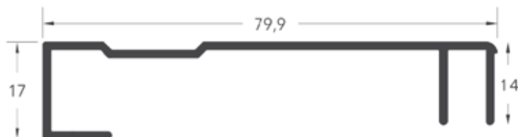
FCX-0212 VISTA INTERNA GIRO
