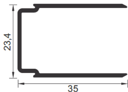
FCX-0228 PROLONGADOR BATENTE
