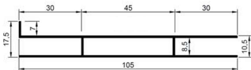
SA-005 VISTA INTERNA
