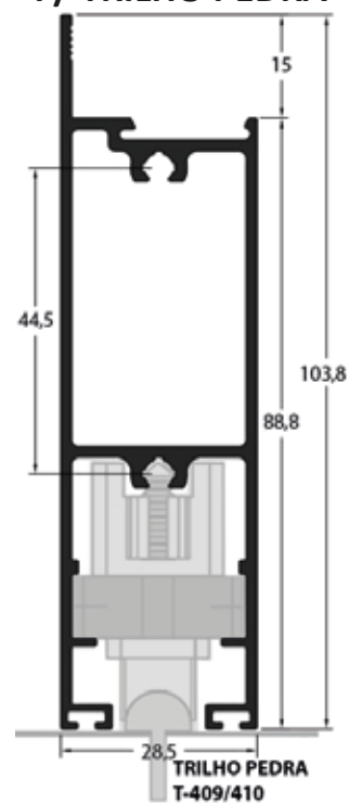
LG-007P P/ TRILHO PEDRA
