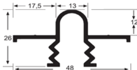
PC-006 TRILHO PORTÃO - CHUMBAR
