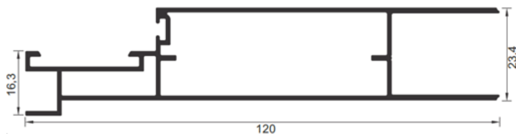
FCX-0211 – BATENTE PIVOTANTE
