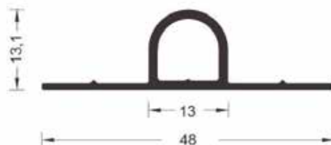
PC-006 TRILHO PORTÃO - CHUMBAR
